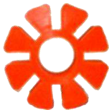
ACOPLE P/BOMBA DE INYECCION CUMMINS. EXT. 3 3/8" INT. 1 1/4" ESP. 1 9/32"
