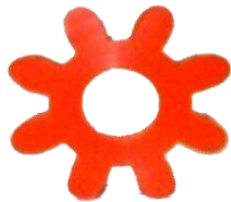
COPLE CHICO DE COMPRESOR PERKINS F-1 EXT. 2 13/16" INT. 15/16" ESP. 23/32"
