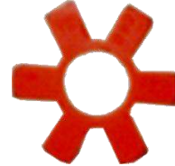
ACOPLE P/BOMBA DE INYECCION CUMMINS/V12 EXT. 2 1/16" INT. 3/4" ESP. 7/16"
