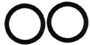
EMPAQUE PARA TAPON DE TANQUE DIESEL OD: 3 11/32" ID: 2 7/16" TK: 3/16"
